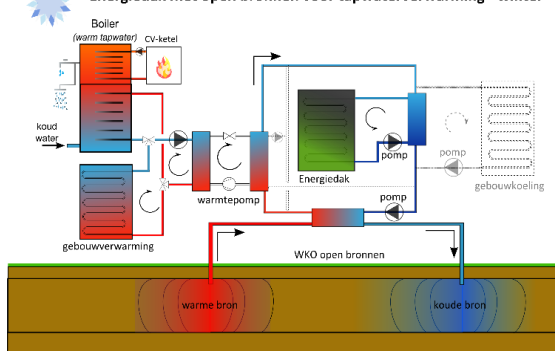
Energiedak met open bronnen voor tapwaterverwarming - winter
